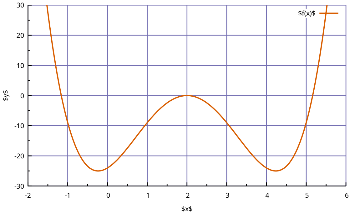
Comportamiento de f(x)=(x-2)^4-10(x-2)^2
